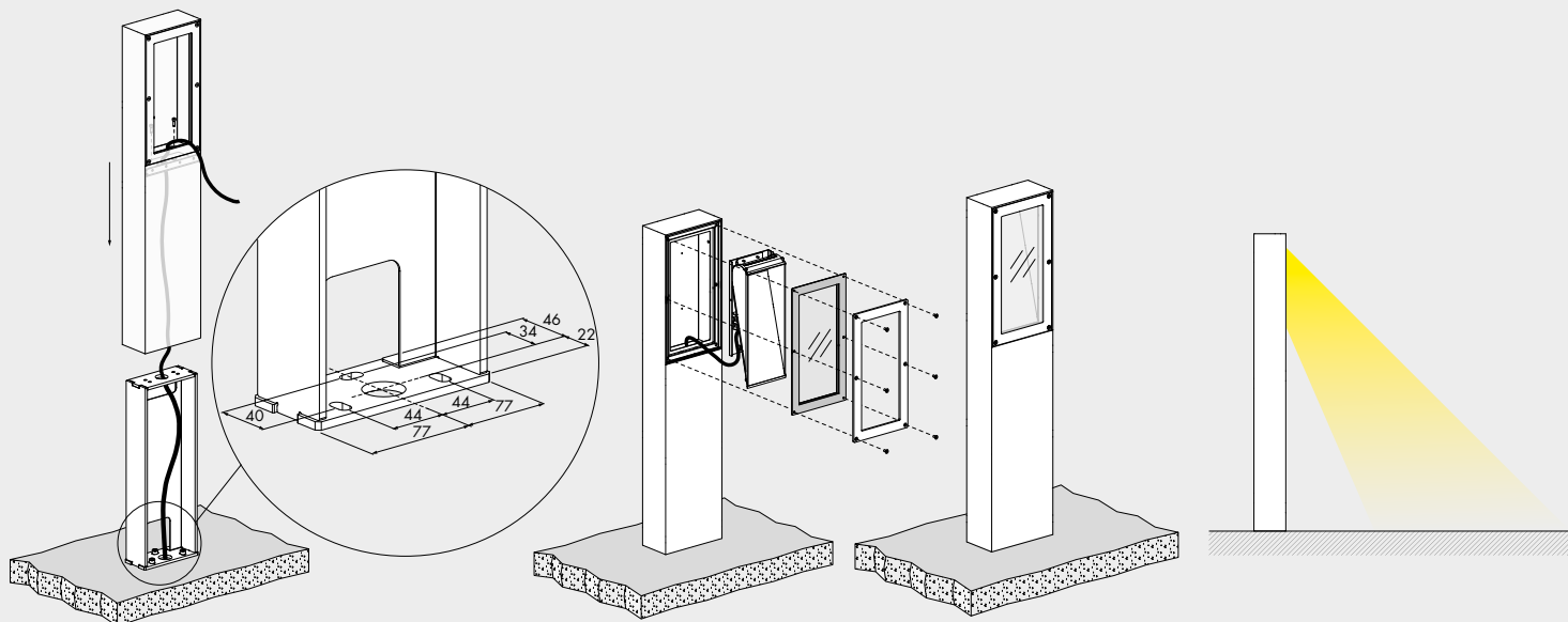
esempio di installazione cubo large palette installation example cubo large palette
